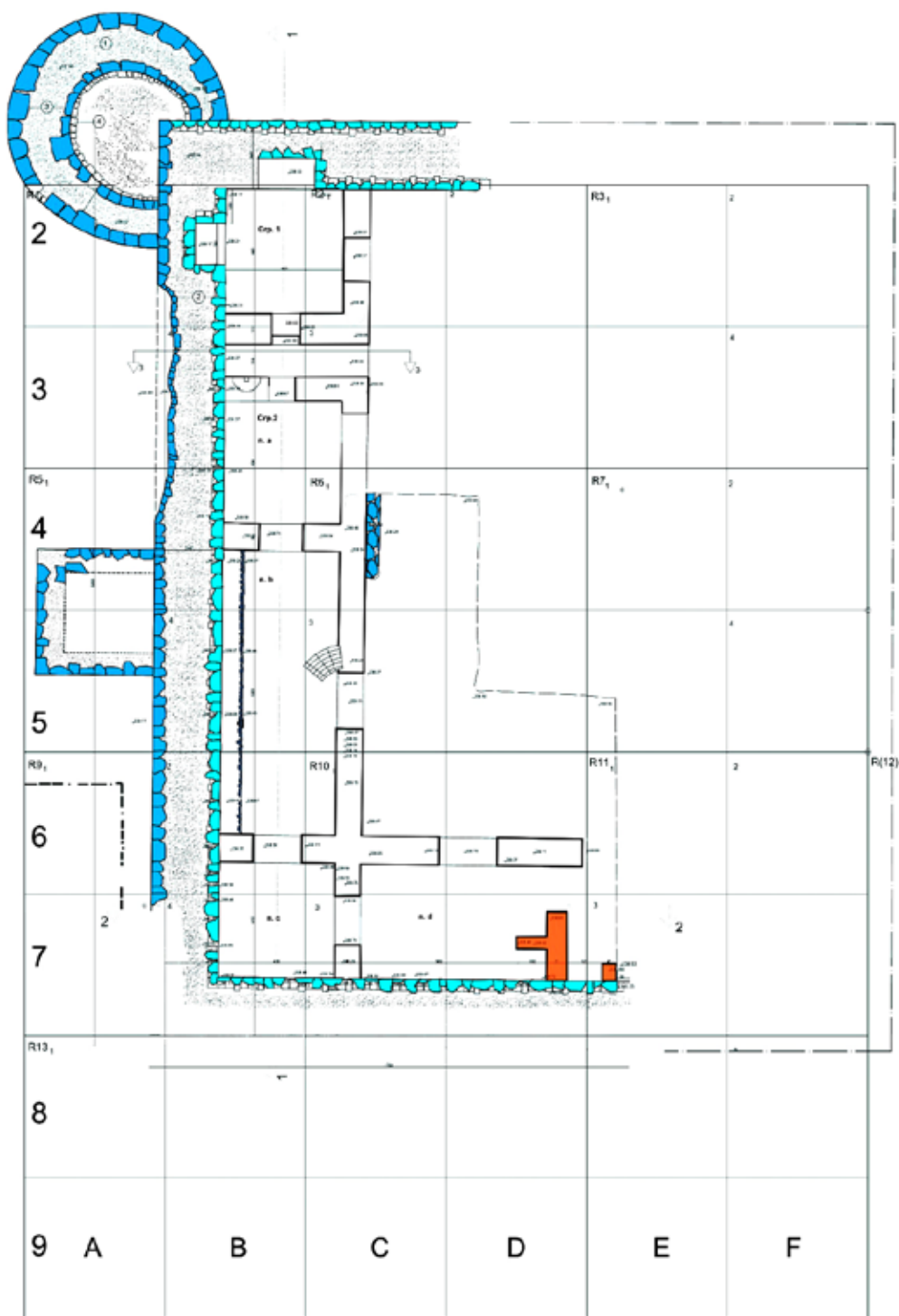
СИТУАЦИОНЕН ПЛАН М 1:50
